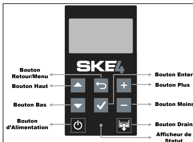
Illustration 43 - Contrôleur SKE4
